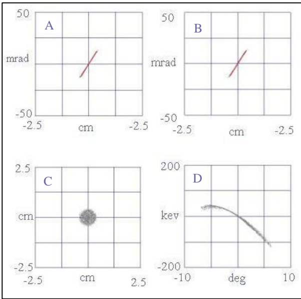
Figure 2 : Trace Space Plots : (A) x-x' (B) y-y' (C) x-y (D) \Delta\Phi-\Delta W .
